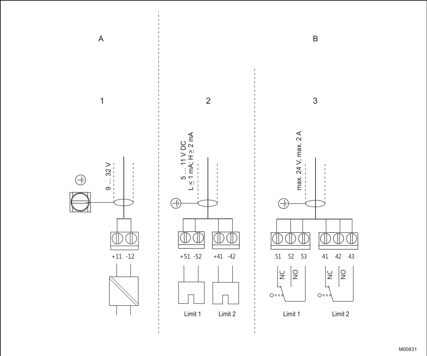
Fig. 7: Empleo de los conductores
