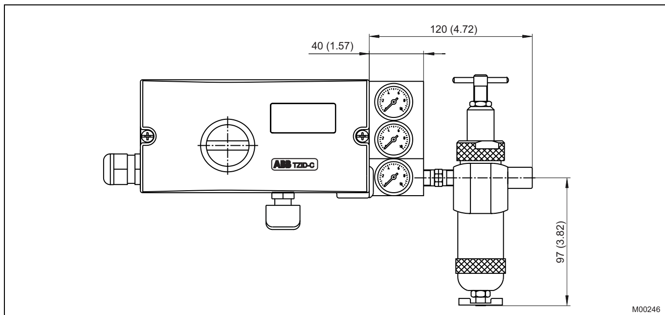
Fig. 12: Regulador de posición TZIDC-110 con bloque de manómetro incorporado y regulador del filtro
