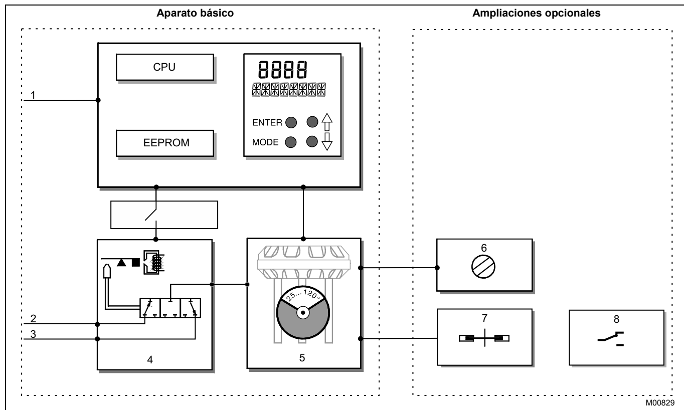
Fig. 1: Representación esquemática del TZIDC-110
