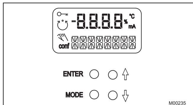
Fig. 4: Elementos de servicio y visualización del TZIDC-110
