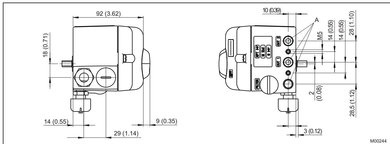
Fig. 10: Vista lateral (de izquierda a derecha) A Conexiones neumáticas, NPT 1/4"-18 o G1/4"
