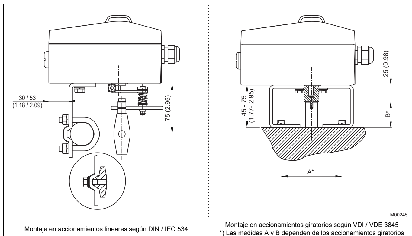
Fig. 11: Dibujo de montaje
