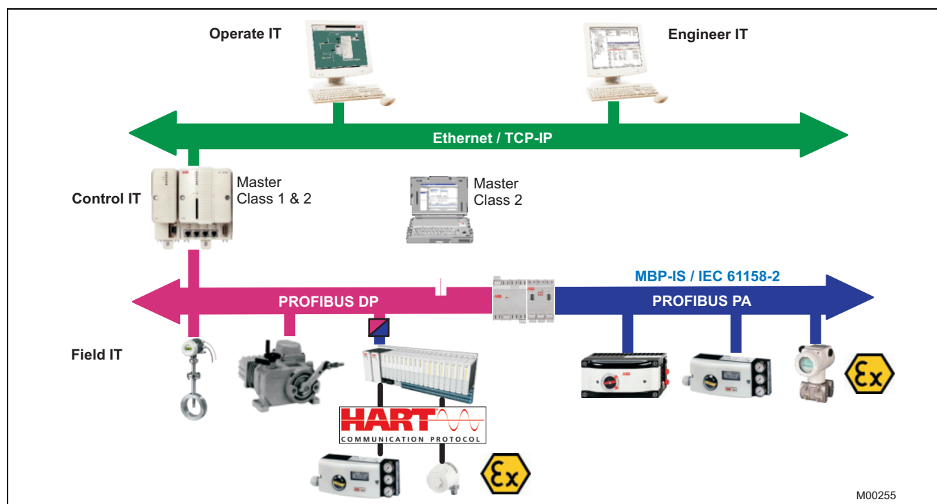
Fig. 5: Comunicación a través de PROFIBUS
