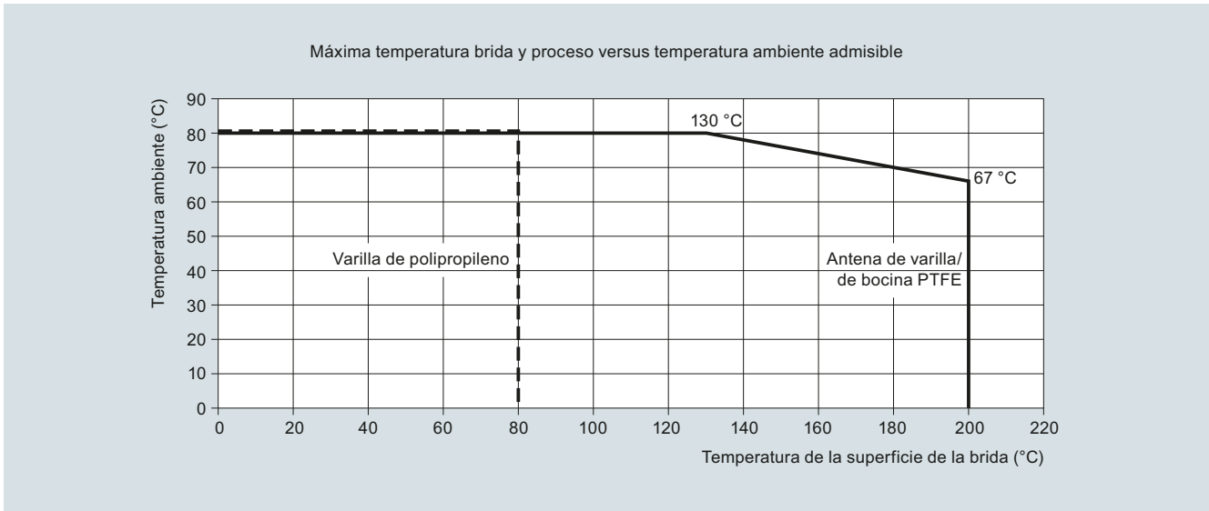
Curva Temperatura ambiente/superficie de la conexión embridada SITRANS LR200
